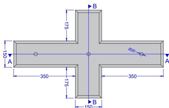
BOVENAANZICHT
