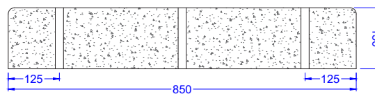
DOORSNEDE B-B
